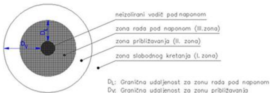
Slika 1. Zona rada pod naponom i zona približavanja
