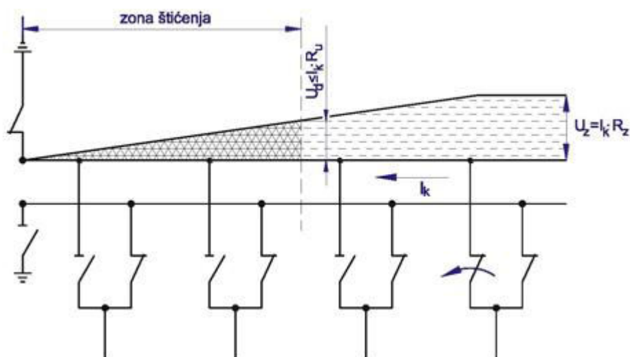
Slika 6. Zona šticećenja uzemljivača
