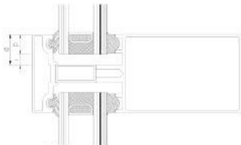
Slika 1 – Ležište stakla u okviru
